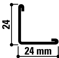
L24x24 C
